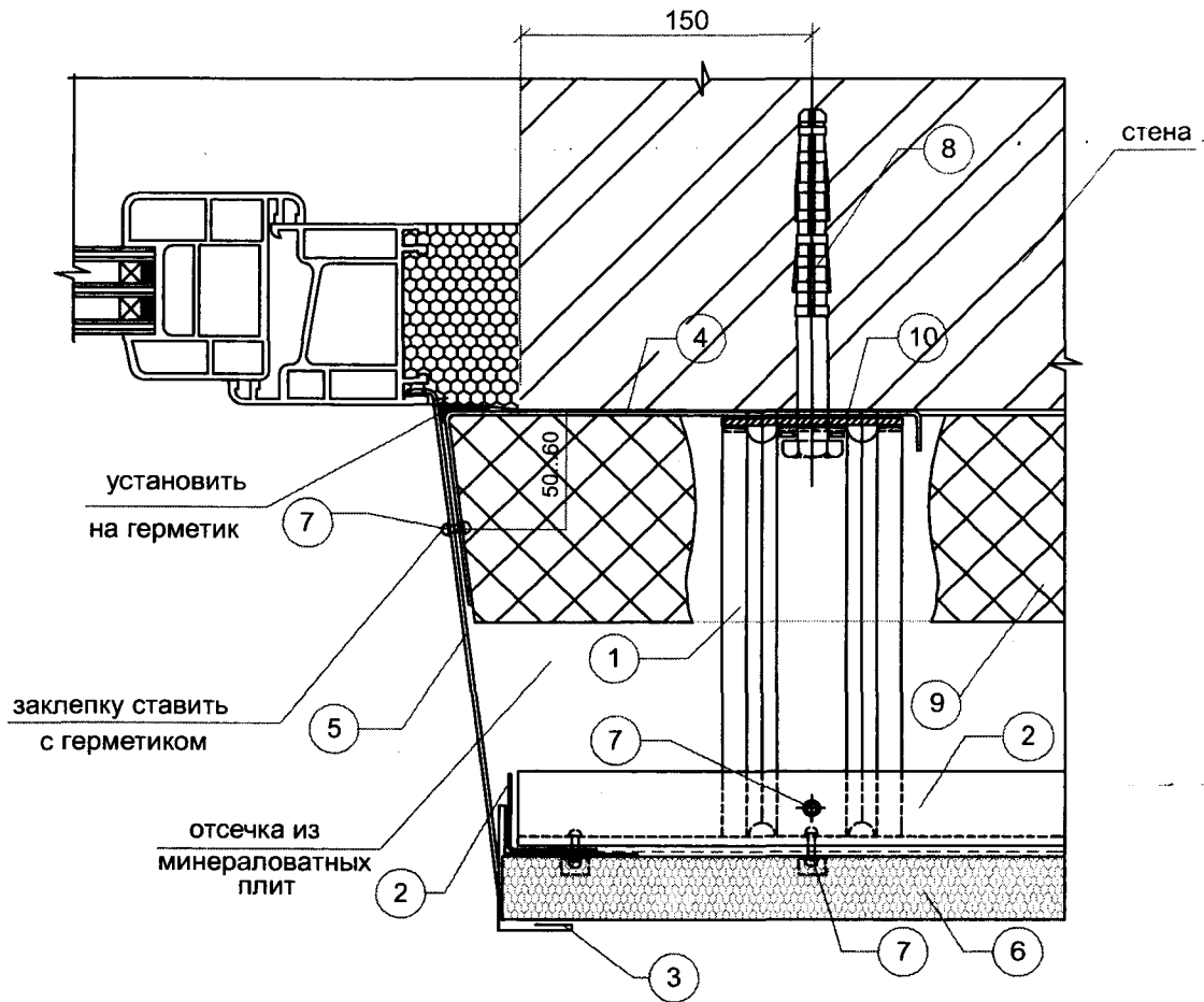
Узел 7. Боковой откос оконного проема
