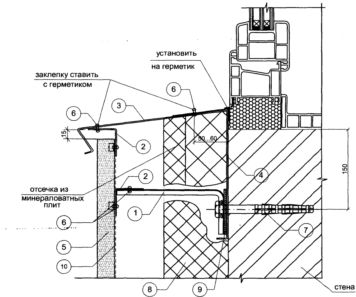
Узел 6. Нижний откос оконного проема
